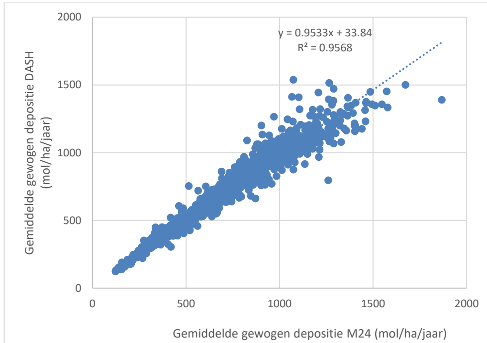
Figuur 3. Gemiddelde gewogen depositie per habitatype per natuurgebied: M24 vs DASH. Vergelijking tussen rekenresultaten van gewogen depositie van DASH met rekenresultaten uit data uit AERIUS Monitor 2024, op basis van dezelfde uitgangspunten (emissiegegevens, rekenjaar, etc.). Gewogen gemiddelde depositieresultaten zijn in mol/ha/jaar.
