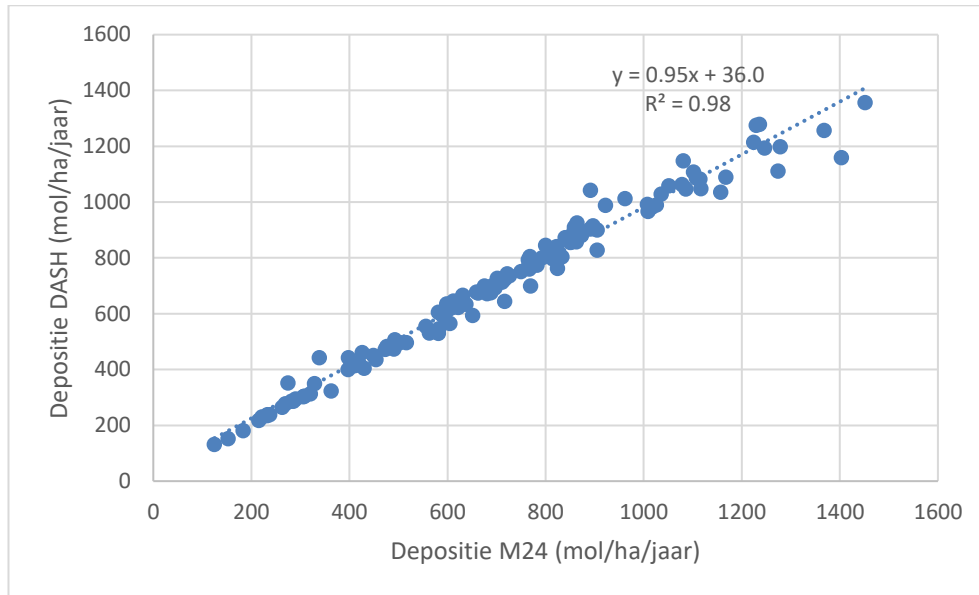
Figuur 2. Gemiddelde gewogen depositie per natuurgebied: M24 vs DASH. Vergelijking tussen rekenresultaten van gewogen depositie van DASH met rekenresultaten uit data uit AERIUS Monitor 2024, op basis van dezelfde uitgangspunten (emissiegegevens, rekenjaar, etc.). Gewogen gemiddelde depositieresultaten zijn in mol/ha/jaar.
